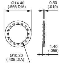
LOCKWASHER
