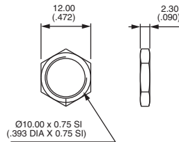
HEX NUT
