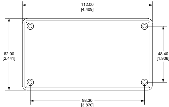
BOTTOM OF LID
