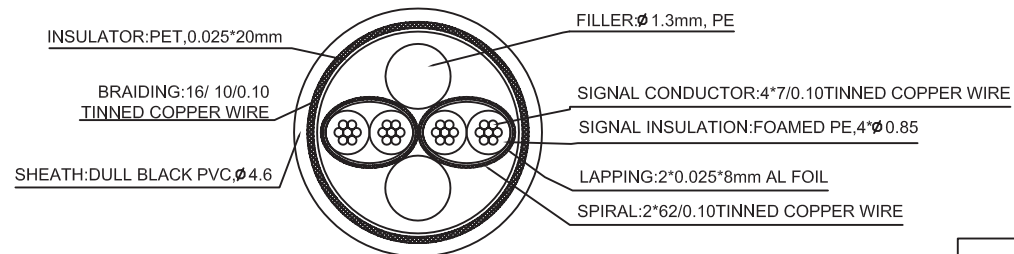
IEEE 1394 4 CORES CABLE
