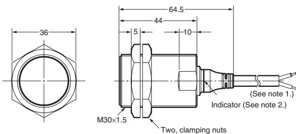
E2A-M30KS10-WP-□□/E2A-S30KS10-WP-□
