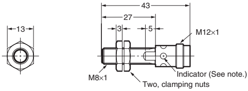
E2A-S08KS01-M1-□□
