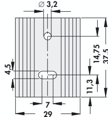
SK 09 37,5 TO 220
