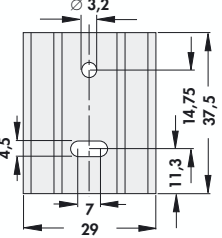
SK 145 37,5 TO 220
