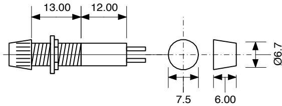
Body Dimensions
