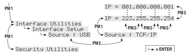
(C) Szczegóły menu UTILITY: Interface Utilities
