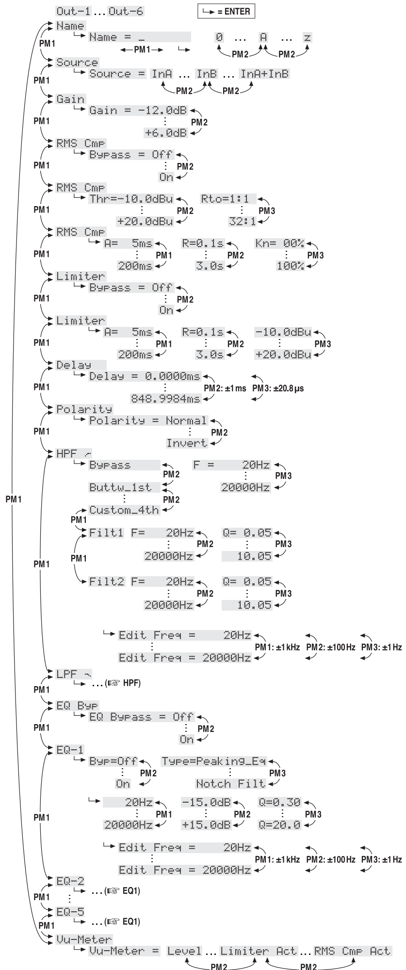
⑦ Estructura del menú para el ajuste de un canal de salida
