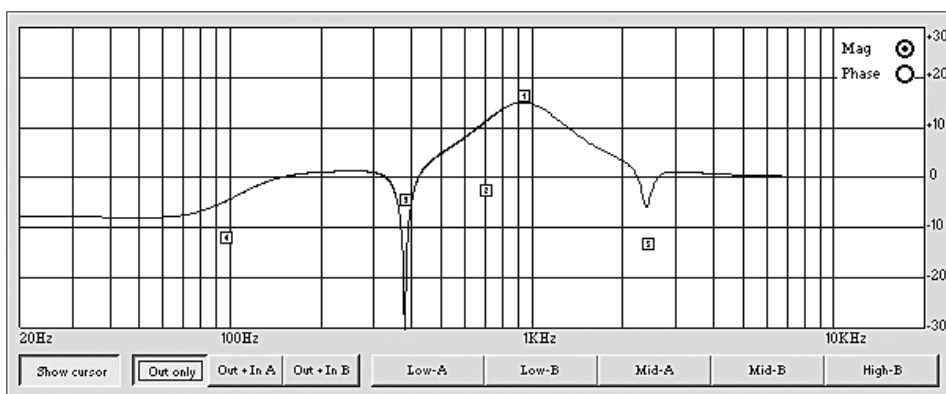
16) Krzywa filtra
