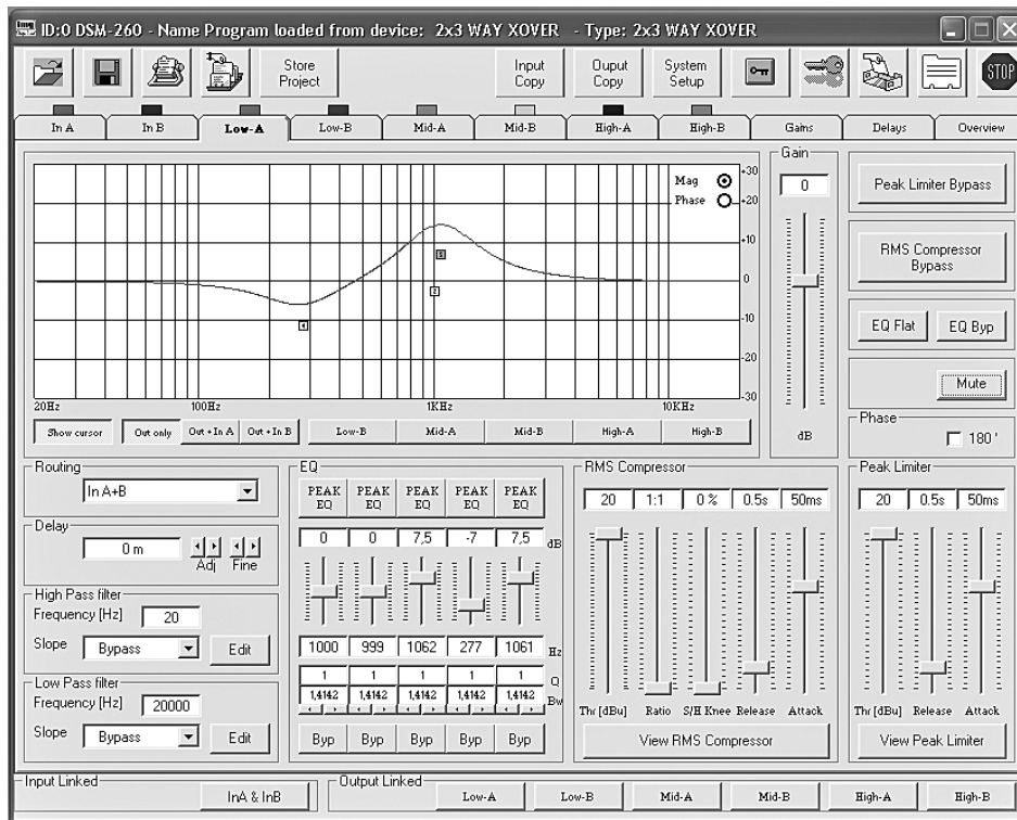
17 Vue canal de sortie "Low-A"
