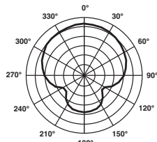
Caractéristique de directivité Caratteristica direzionale
