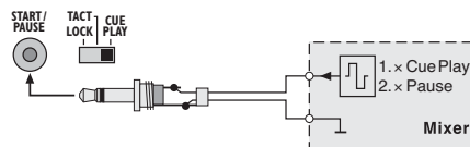
Fig. 10 Avviamento con fader tramite un impulso
