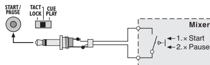
Fig. 9 Avviamento con fader tramite un pulsante
