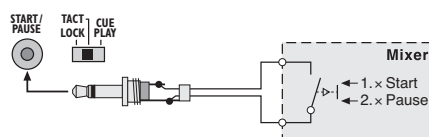
Rys. 9 Funkcja fader start sterowana przełącznikiem chwilowym
