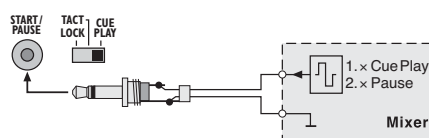
Rys. 10 Funkcja fader start sterowana impulsem
