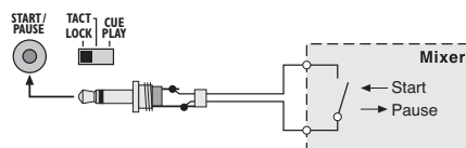
Schéma 8 démarrage électrique via un interrupteur marche/arrêt
