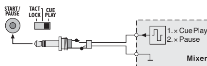
Figuur 10 Faderstart via stuurimpuls
