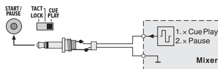
Schéma 10 démarrage électrique via une impulsion de commande
