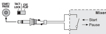
Abb. 8 Faderstart über Ein-/Ausschalter
