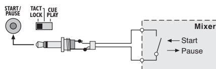
Fig. 8 Inicio Fader mediante un interruptor ON/OFF
