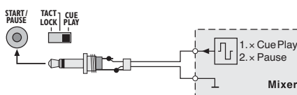
Abb. 10 Faderstart über Steuerimpuls
