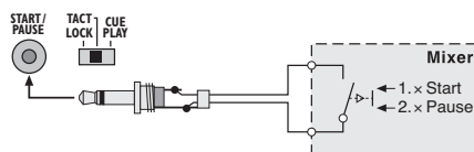
Fig. 9 Inicio Fader mediante un pulsador
