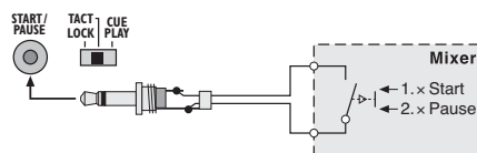
Schéma 9 démarrage électrique via un bouton poussoir momentané
