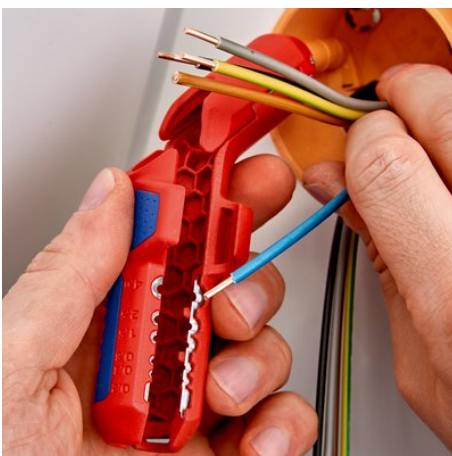
Afisolering af enkelte ledere
