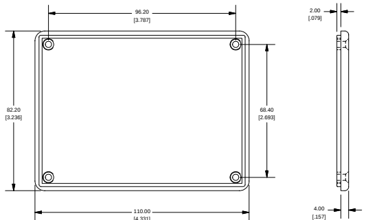
BOTTOM OF LID
