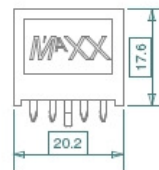
H1810-2x4
