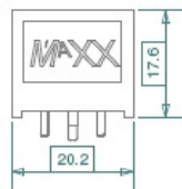
H1810-2x1
