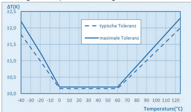
Abbildung 2 Typische und maximale Toleranz der Temperaturmessung
