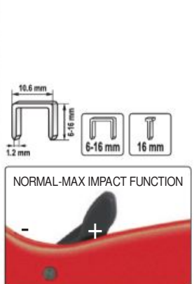
YATO staples size / rozmiar zszywki (mm) YT-7005 10.6x6.0-16.0x1.2 6/24
