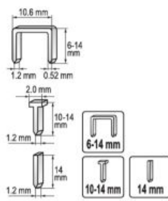
YATO YT-7003 6/24
